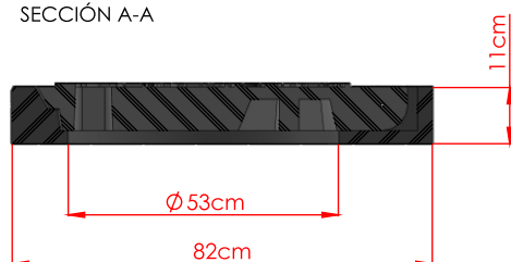
SECCIÓN A-A
